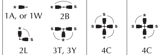
Photocell Receptacle
